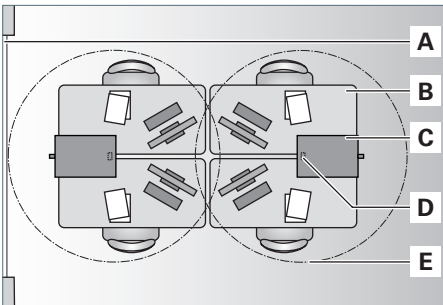
Fig. 8: Apparecchio d'illuminazione con più di 8000 lm (DPS 288, DPT 288).
