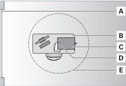
Fig. 7: Apparecchio d'illuminazione fino a 6000 lm (DPS 240, DPT 240).
