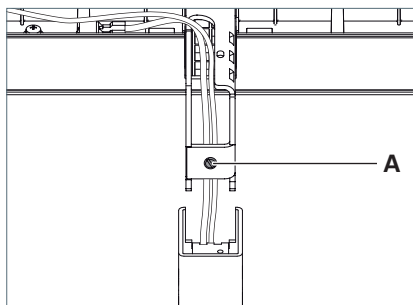
Fig. 16: Regolazione della testa dell'apparecchio d'illuminazione.
