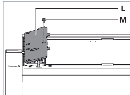
Fig. 6: Abdeckung montieren.
